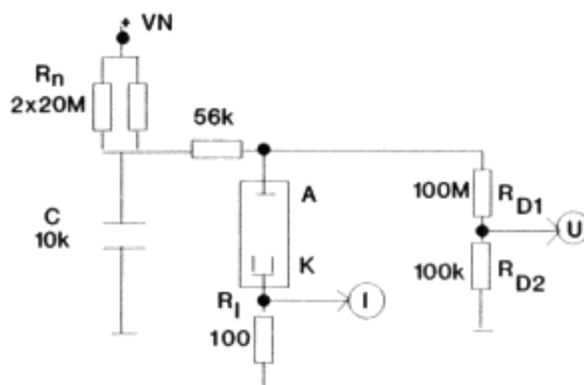
Obr. 1: Elektrické schéma zapojení napájecího zdroje He-Ne laseru pro provoz v impulzním režimu.
